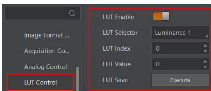
图12-23 LUT 设置
