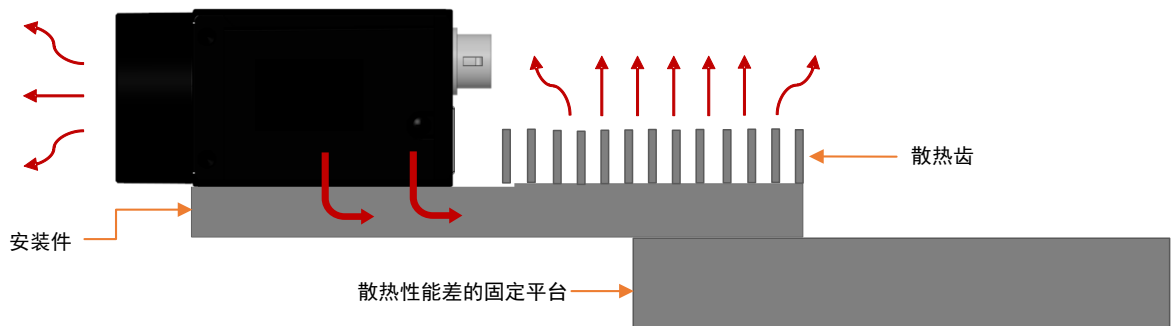
图4-14 增加散热齿的安装件
