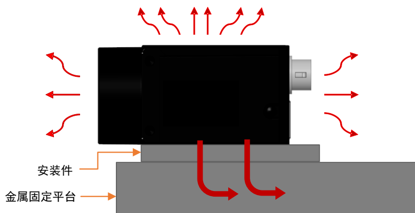
图4-12 安装件散热
