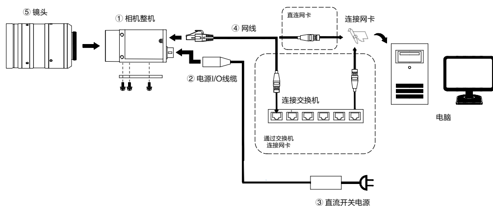
图6-2 整机连接
