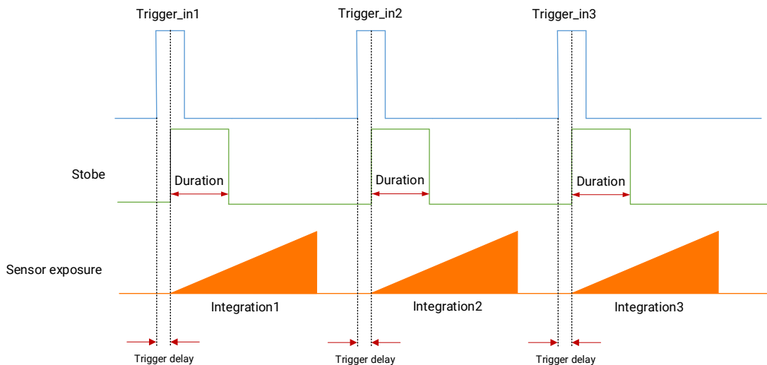
图8-26 Strobe 持续时间时序
