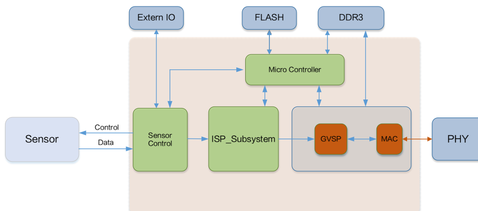
图3-1 工作原理
