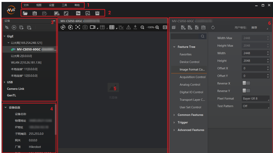
图6-10 软件主界面
