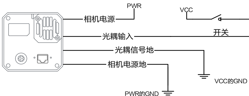
图7-10 Line 0 接开关
