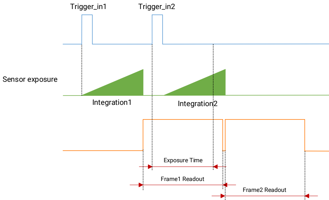
图8-16 第2帧曝光移动处理时序
