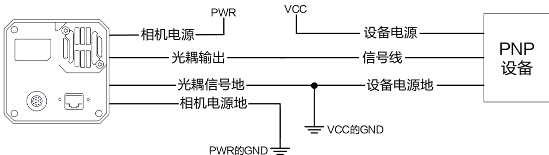
图7-11 Line 1 接 PNP 设备
