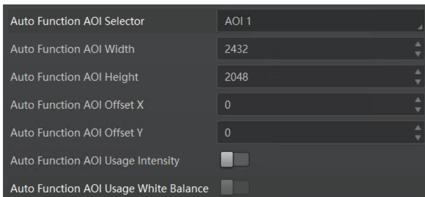
图12-6 AOI 功能
