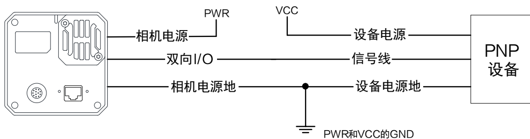
图7-16 Line 2 作为输出接 PNP 设备
