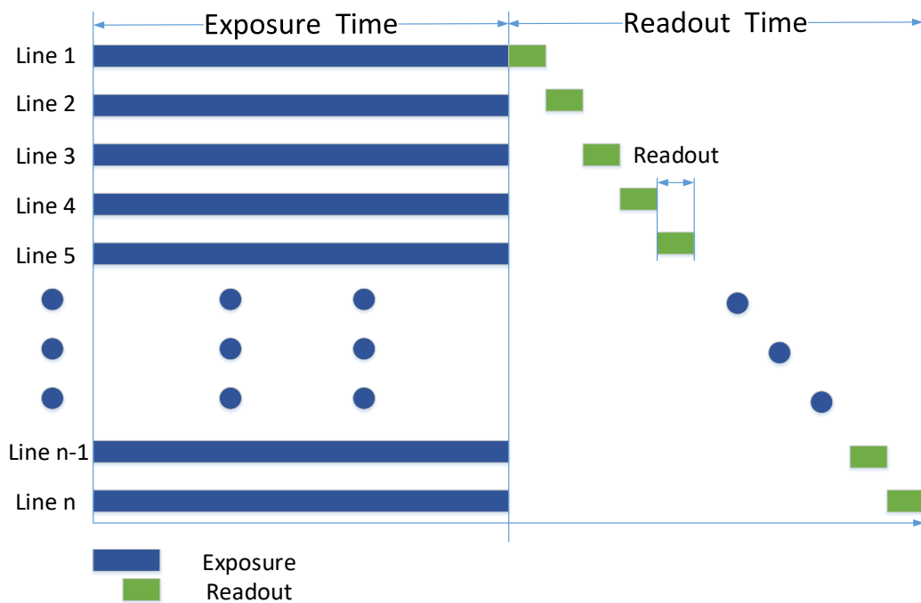
图9-1 全局快门
